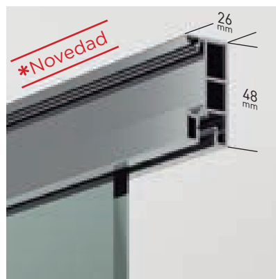
Nuevo perfil superior y nueva fijación del vidrio fijo.
