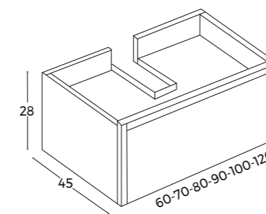
MUEBLE SUSPENDIDO UN CAJÓN CON SALVASIFÓN
